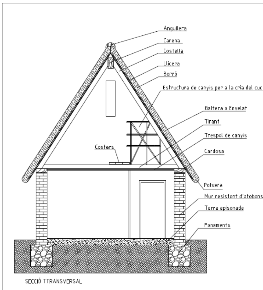
Secció transversal barraca d'horta. Vivenda. Delineació de l'autor.
