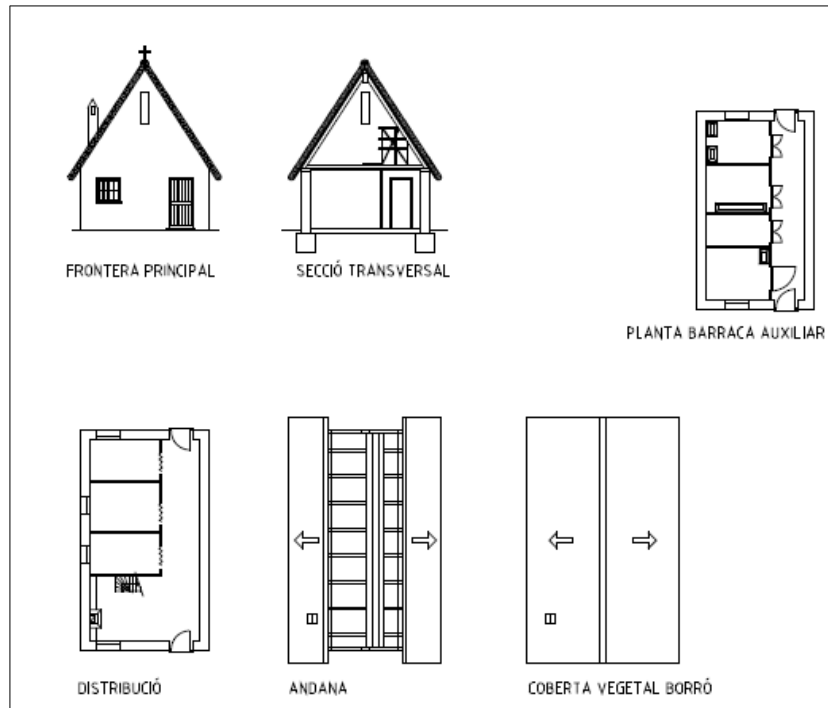
Plantes, frontera i secció d'una barraca d'horta. Delineació de l'autor.
