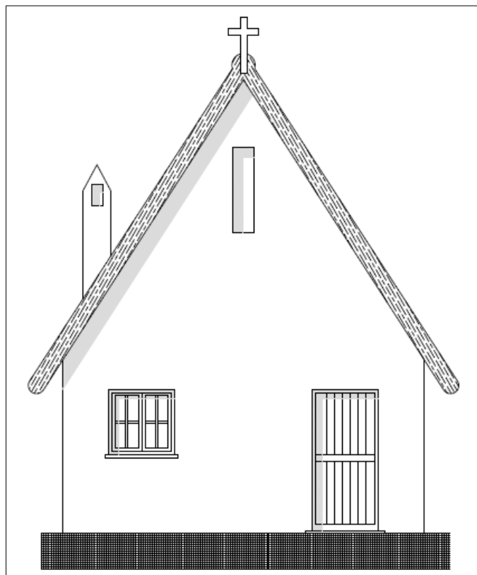
Frontera principal barraca d'horta. Vivenda. Delineació de l'autor.
