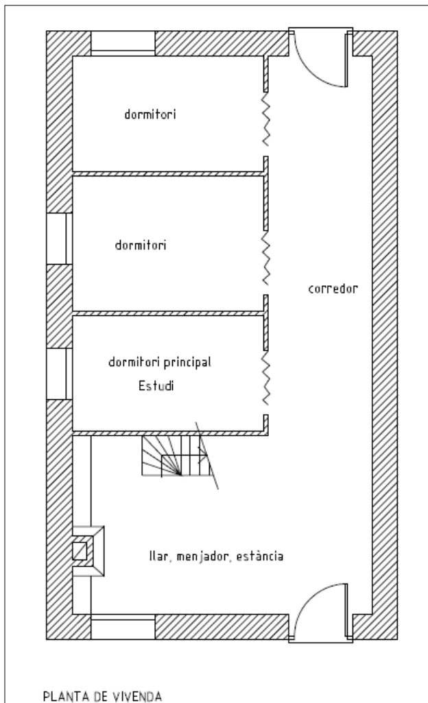
Planta de distribució barraca d'horta. Vivenda. Delineació de l'autor.
